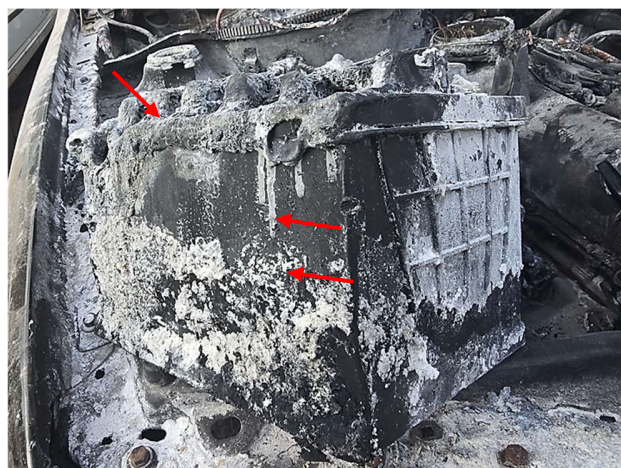
Figuras 48 e 49 – Setas vermelhas mostram bateria apresentando anormalidades técnicas por escorrimento de material eletrólito, devido ao aquecimento interno. Fonte: Acervo pessoal.
