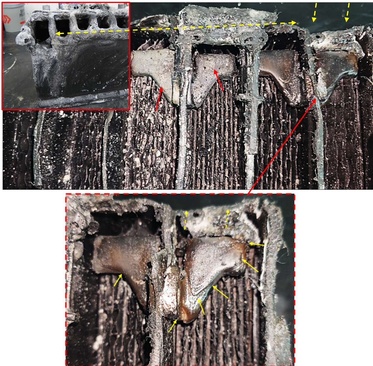
Figura 52 – Setas vermelhas mostram conectores das células sem anormalidades técnicas. Setas amarelas tracejadas mostram derretimento da carcaça. Setas amarelas mostram conector positivo apresentando anormalidades técnicas por superaquecimento, modificando as propriedades físico-químicas da estrutura. Fonte: Acervo pessoal.
