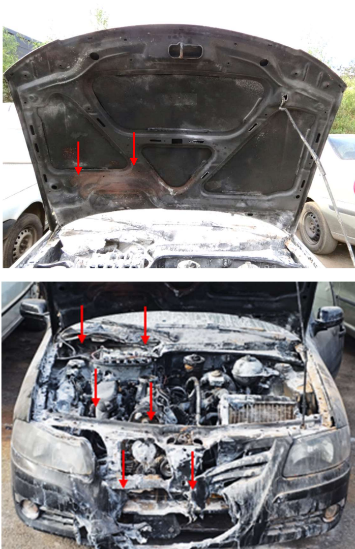
Figuras 42 e 43 - Setas vermelhas mostram motor com danos por queima e concentração do lado direito, com orientação de trás para frente. Fonte: Acervo pessoal.
