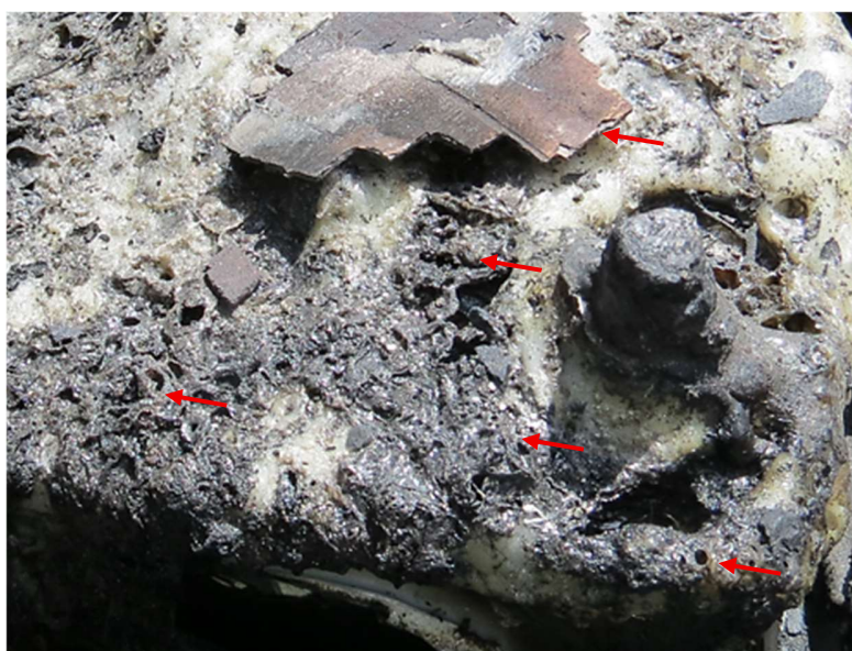
Figuras 34 e 35 - Mostram parte externa das baterias com danos por queima interna e formação de microfuros, em decorrência da reação química e formação interna de gases inflamáveis (hidrogênio). Fonte: Acervo pessoal.
