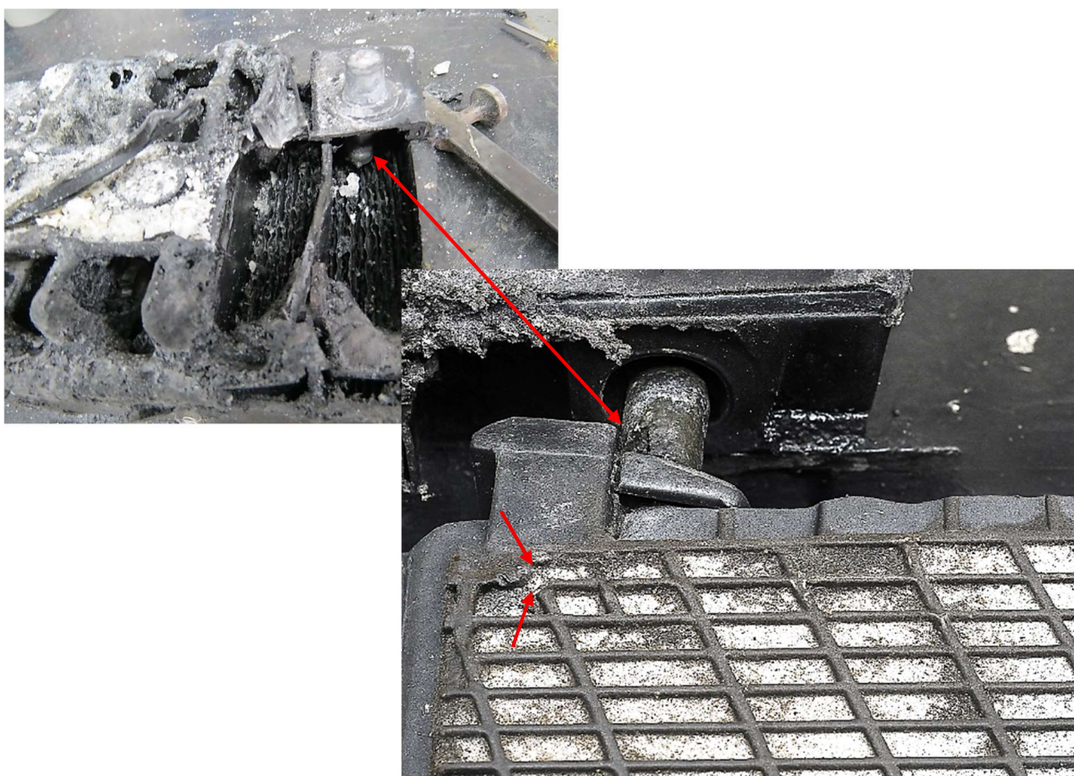
Figuras 53 e 54 – Setas vermelhas mostram vaso/placa positiva da bateria apresentando anormalidades técnicas por ruptura na parte interna e ausência/ressecamento do material eletrolítico. Fonte: Acervo pessoal.
