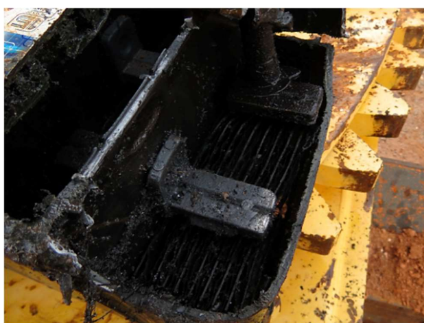
Figuras 64 e 65 - Fragmentação da placa negativa de chumbo, o que promove o curto-circuito interno. Fonte: Acervo pessoal.
