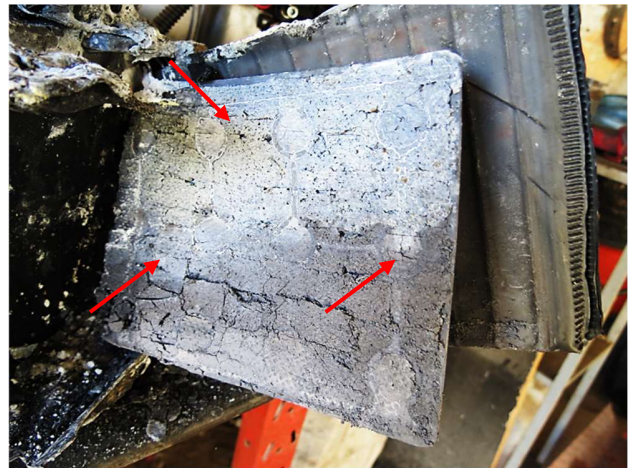
Figuras 68 e 69 - Formação de cristais de sulfato de chumbo em placas internas, indicando sulfatação avançada e curto-circuito. Fonte: Acervo pessoal.
