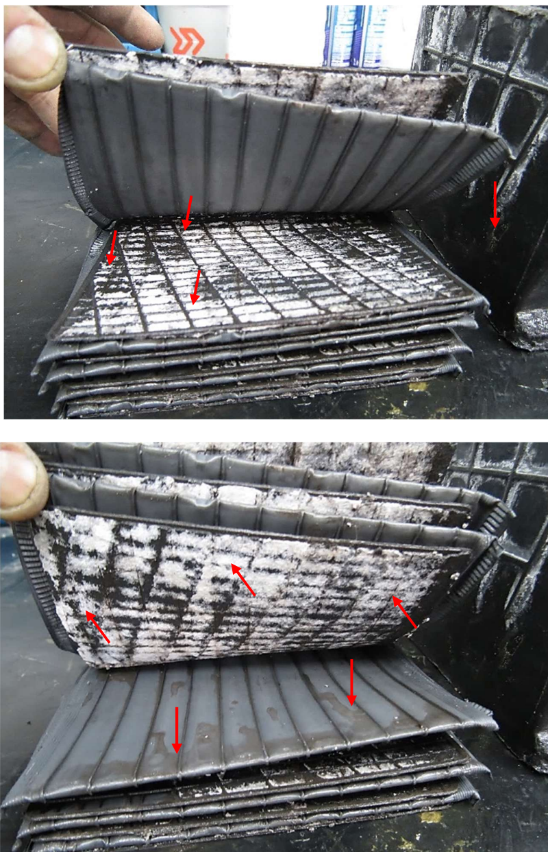
Figura 55 e 56 – Setas vermelhas mostram vaso/placa positiva da bateria apresentando anormalidades técnicas por formação de material esbranquiçado (sulfato de chumbo).
